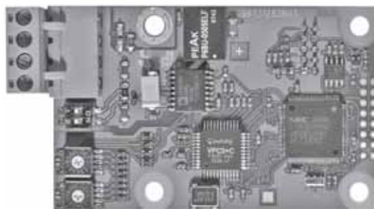
Fig. 106 Grundfos CIM communication interface module
