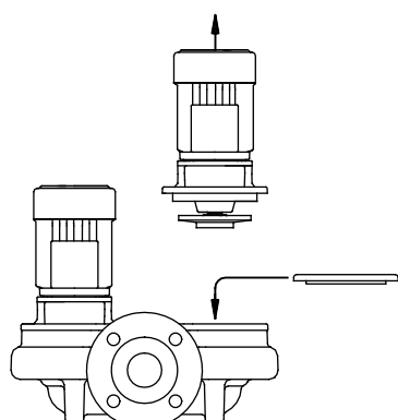
Fig. 97 Blanking flange
